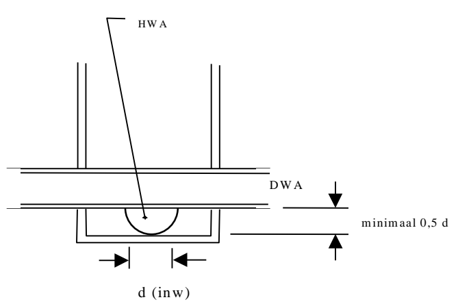
Doorsnede B
