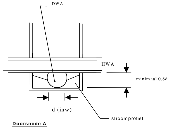
Doorsnede A
